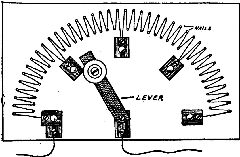
Fig. 314.—A Rheostat.
